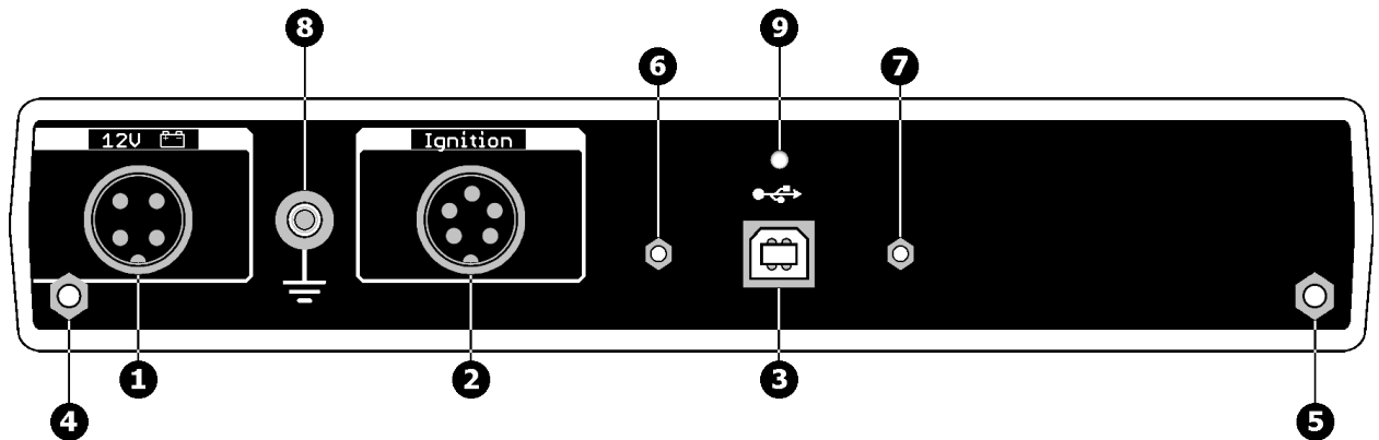
Задняя панель USB Autoscope IV.
