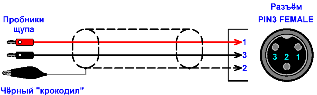
Схема распиновки дифференциального осциллографического щупа.
