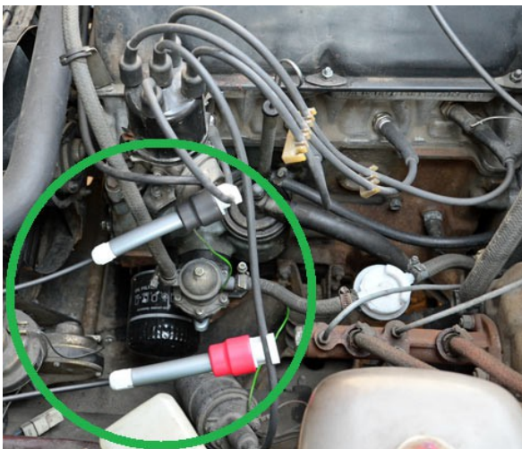
Правильное расположение кабелей ёмкостных датчиков.
